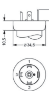
ISO 4400 (IP 65)
