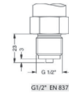
G1/2" EN 837
